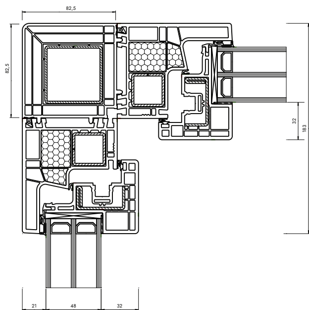
Accoppiamento 90 gradi
